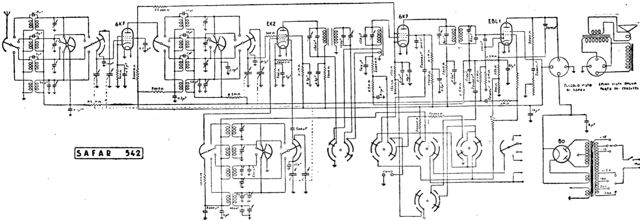
RADIO SAFAR. — Mod. 542 e 542 R. — Produzione 1938-39. — Media frequenza: 448 kHz. Gamme: cc. (95-19 MHz.), c. (55-10 MHz.), m. (520-1500 kHz.), l. (140-300 kHz.).
